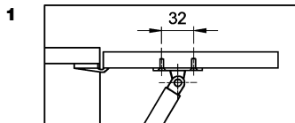
621 - Attacco per anta in legno
