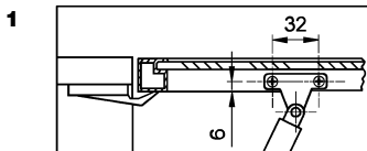
621 AL - Attacco per anta in alluminio
